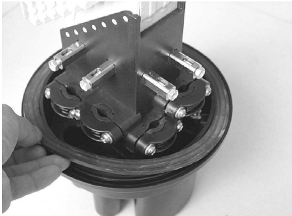
Элементы фиксации оптического кабеля внутри муфты
