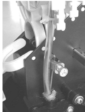
Элементы фиксации оптического кабеля внутри муфты
